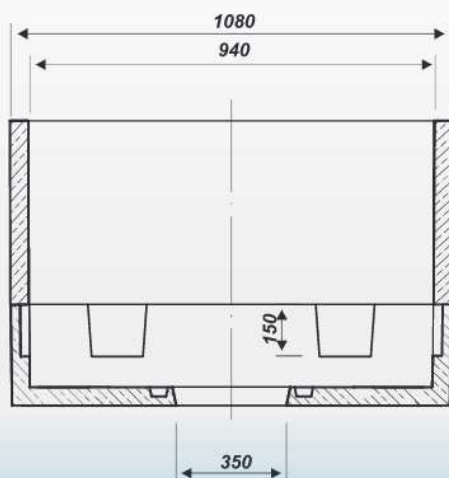
Przekrój podłużny
