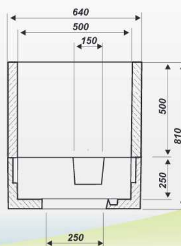
Przekrój poprzeczny
